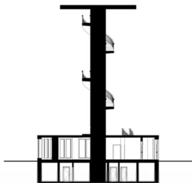
ŘEZ OBJEKTEM
