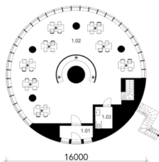
PŮDORYS KAVÁRNY (1.NP)
