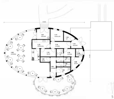
PŮDORYS 1.NP 1:150
