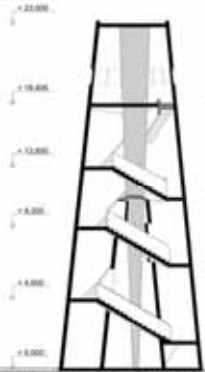
ŘEZ A-A' - ROZHLEDNA M 1:150
